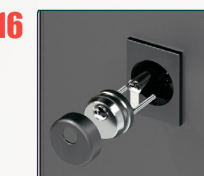
DEFENDER (PROTECTOR CILINDRU) DIN OTEL CARBONITRURAT — 60 HRC
