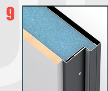
IZOLAȚIE TERMICĂ INTERNĂ — POLISTIREN, GROSIME 70 MM, DENSITATE 35 KG/M³ 70 MM, DENSITATE 35 KG/M³
